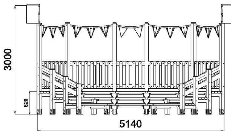
VISTA LATERALE
