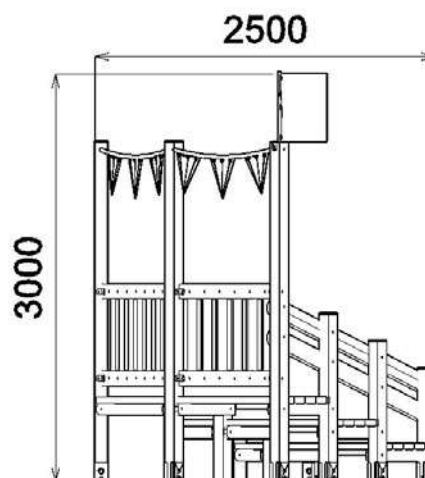
VISTA LATERALE
